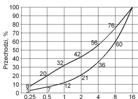
Rysunek 1. Krzywe graniczne uziarnienia kruszywa do betonu
