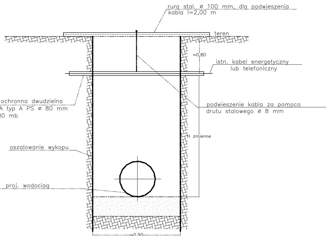
PRZEKROJ A-A
