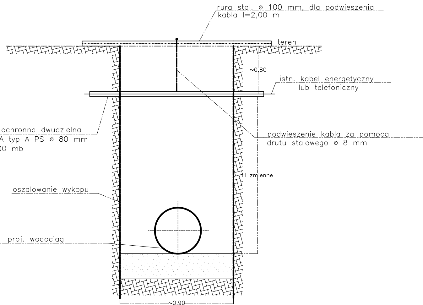
PRZEKROJ A-A
