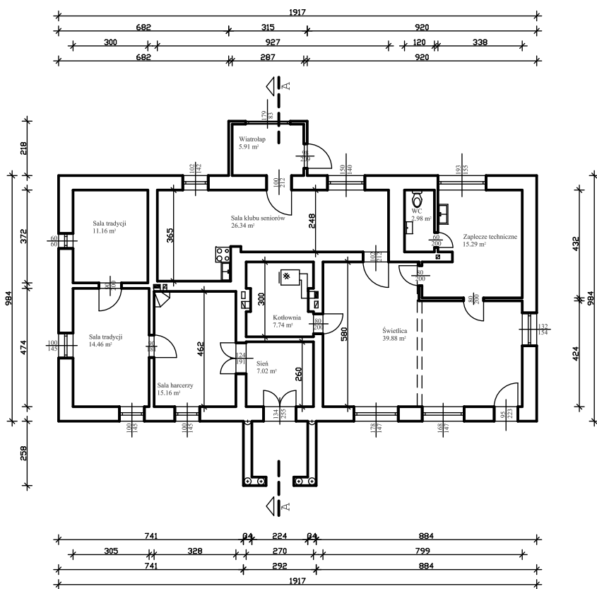
INWENTARYZACJA PRZYZIEMIE 1:100
