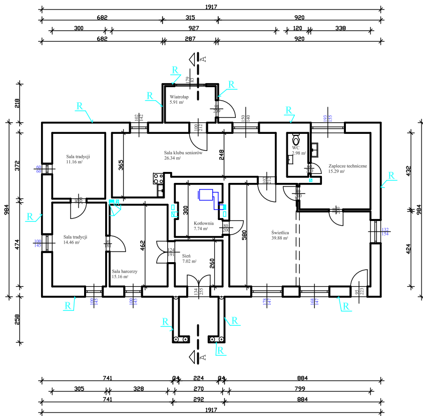
PRZYZIEMIE 1:100
