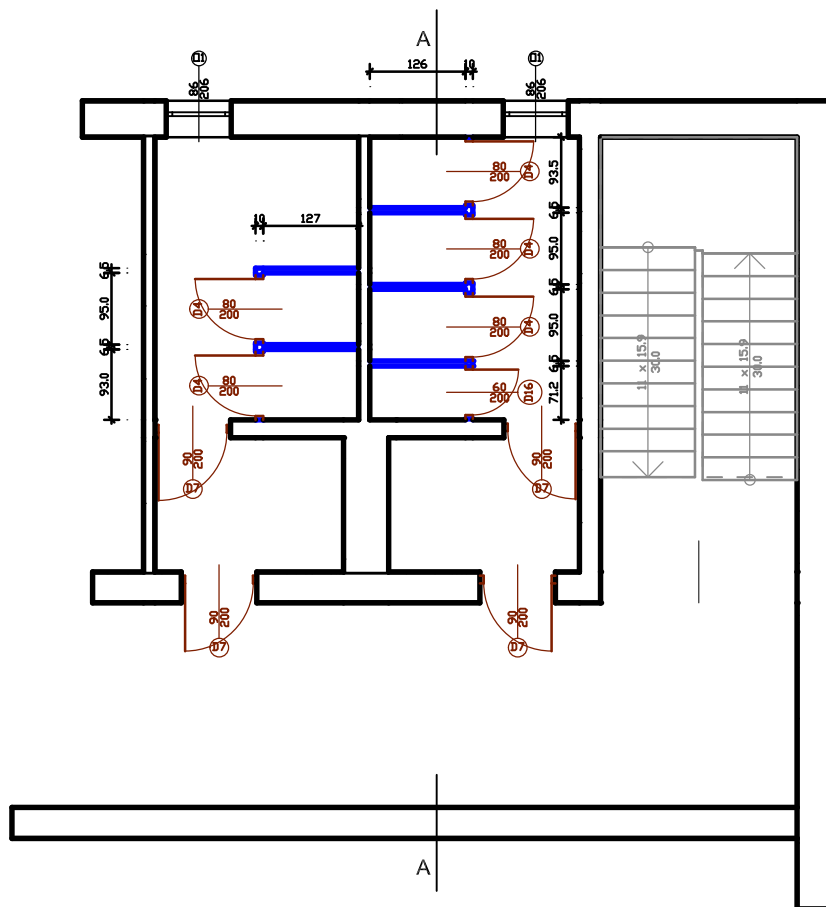
RZUT KONDYGNACJI POWTARZALNEJ WĘZŁA SANITARNEGO
