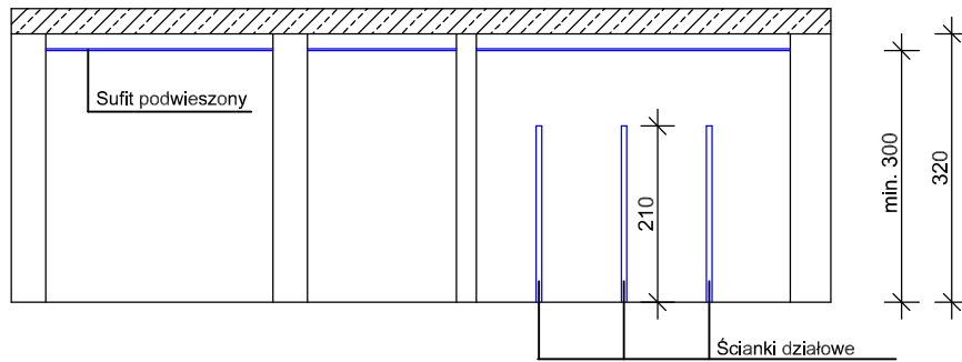
PRZEKRÓJ A-A 1:100
