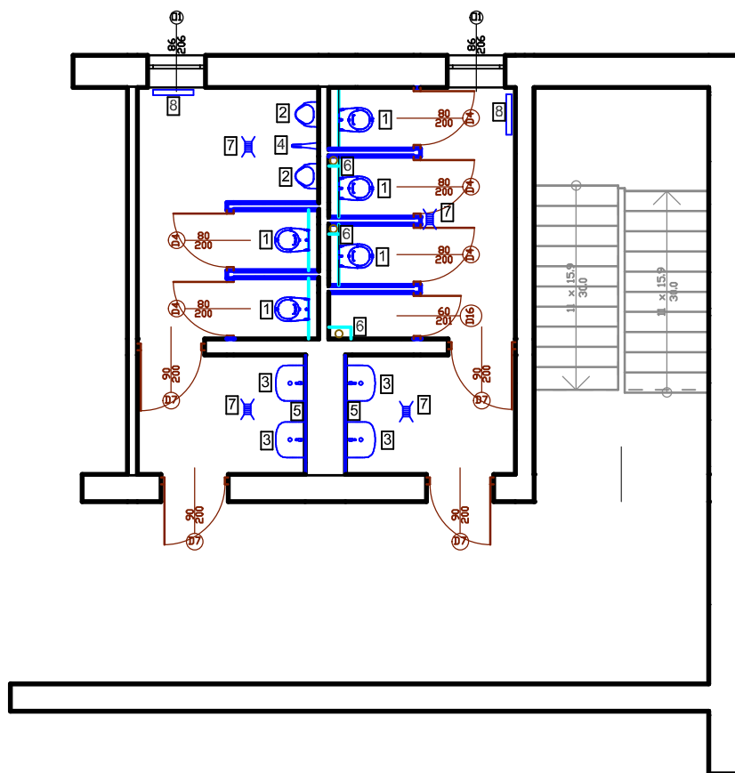
RZUT KONDYGNACJI POWTARZALNEJ WĘZŁA SANITARNEGO
